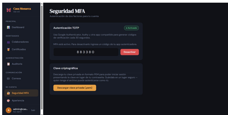
Figura 14: desactivación autenticación multifactor - paso 2
